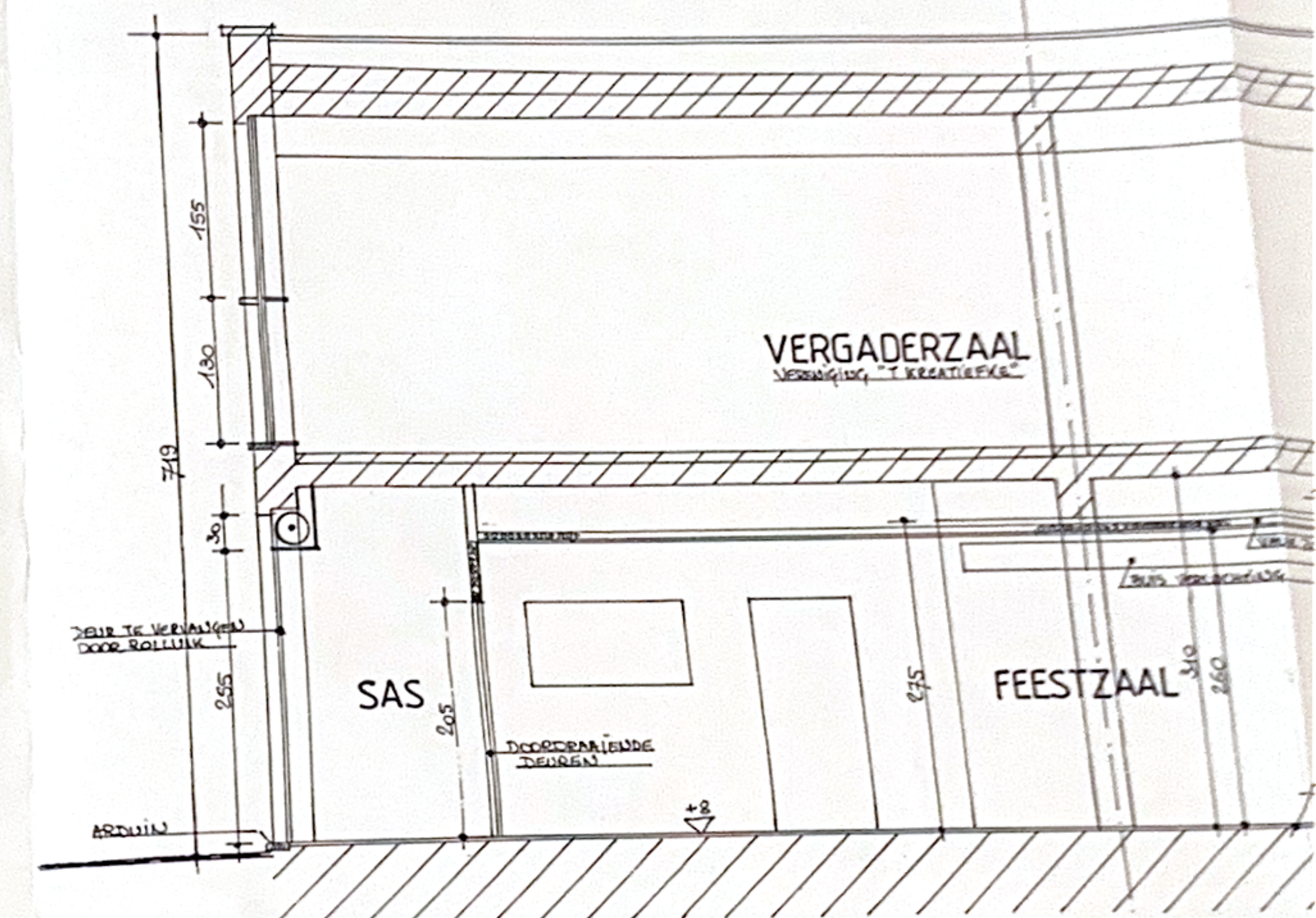
DOORSNEDE AA
