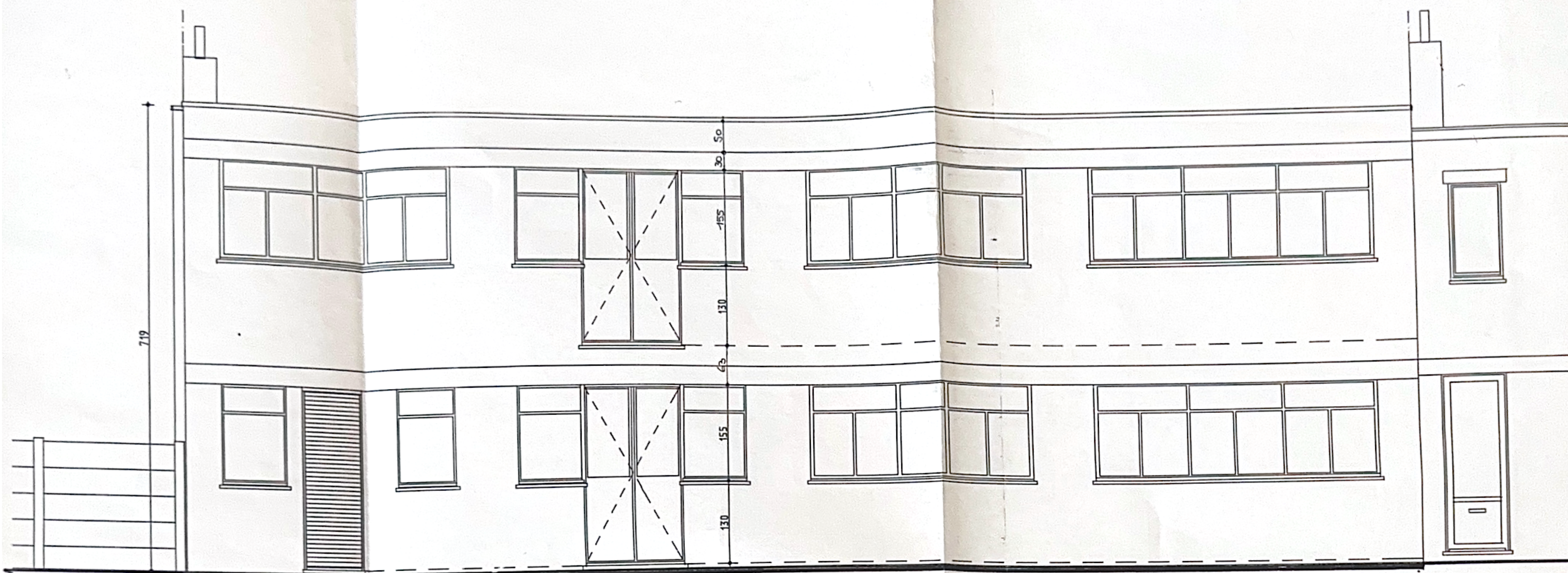
GEVEL bestaat 1/50
